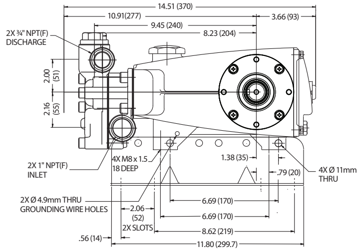
Modelle 1540E, 1540EC, 1541, 1541C
